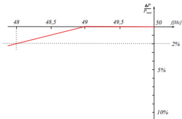
Joonis 2 – Maksimumvõimsuse vähenemine sageduse vähenemisel
